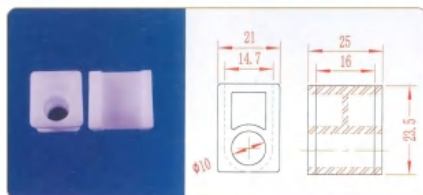
品名: 下插件 材质: PE
