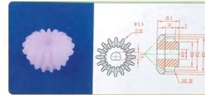
品名: 一体组合齿轮 规格: 16Z伞+16Z直×23L 材质: PVDF 编号: CT-ZHCL-010
