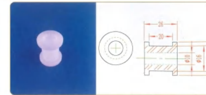
品名: Φ10轴套 规格: Φ10×26L 材质: UPE 编号: CT-ZT-012
