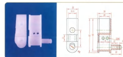
品名: 35插件 材质: PVDF
