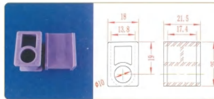
品名: 30上插件 材质: PE
