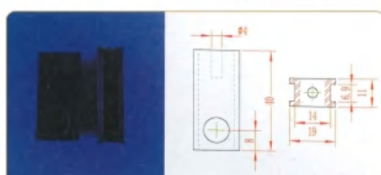
品名: 45下插件 材质: MC
