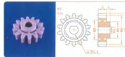
品名: 14齿42直齿轮 规格: M3×14Z 材质: PP 编号: CT-ZCL-074
