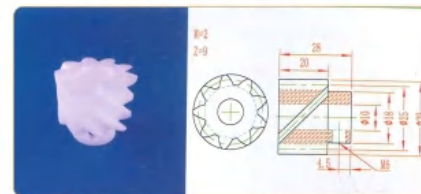
品名: 9齿螺旋齿轮 规格: M2×9Z×28L 材质: UPE 编号: CT-LXCL-009
