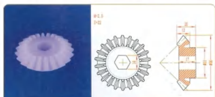
品名: 22齿伞齿轮 规格: M3×22Z×20L 材质: PVDF 编号: CT-SCL-039
