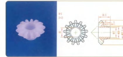
品名: 13齿伞齿轮 规格: M3×13Z×20.5L 材质: PVDF 编号: CT-SCL-002
