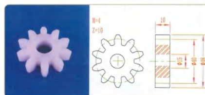
品名: 10齿43直齿轮 规格: M4×10Z 材质: PE 编号: CT-ZCL-077
