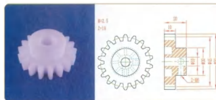
品名: 18齿45直齿轮 规格: M2.5×18Z 材质: PP 编号: CT-ZCL-082
