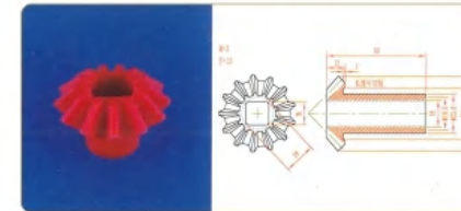
品名: 13齿伞齿轮 规格: M3×13Z×50L 材质: PVDF 编号: CT-SCL-006
