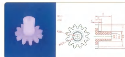
品名: 12齿40直齿轮 规格: M3.3×12Z 材质: PVDF 编号: CT-ZCL-051
