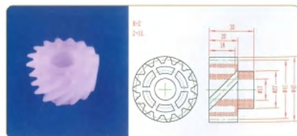
品名: 15齿螺旋齿轮 规格: M2×15Z×33L 材质: UPE 编号: CT-LXCL-071
