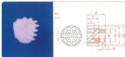
品名: 10齿螺旋齿轮 规格: M2×10Z×28L 材质: PVDF 编号: CT-LXCL-014
