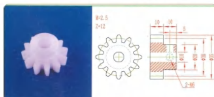
品名: 12齿30直齿轮 规格: M2.5×10Z 材质: PP 编号: CT-ZCL-027
