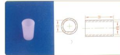
品名: \Phi 16 轴套 规格: \Phi 16D15 \times 39L 材质: PVDF 编号: CT-ZT-032
