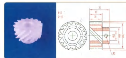
品名: 16齿40直齿轮 规格: M2.5×16Z 材质: PP 编号: CT-ZCL-069
