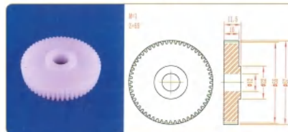
品名: 55齿55直齿轮 规格: M1×55Z 材质: PP 编号: CT-ZCL-106
