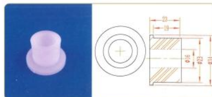
品名: \Phi 16 轴套 规格: \Phi 16 \times 23L 材质: PE 编号: CT-ZT-030
