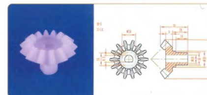
品名: 14齿伞齿轮 规格: M3×14Z×32L 材质: PVDF 编号: CT-SCL-009
