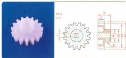
品名: 16齿40直齿轮 规格: M2.5×16Z 材质: PP 编号: CT-ZCL-066
