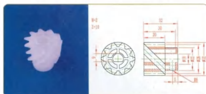
品名: 10齿螺旋齿轮 规格: M2×10Z×32L 材质: PVDF 编号: CT-LXCL-019
