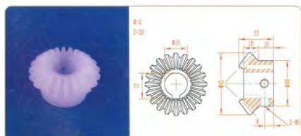
品名: 20齿伞齿轮 规格: M2×20Z×23L 材质: PVDF 编号: CT-SCL-037
