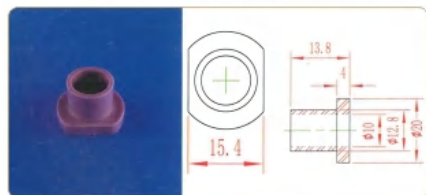
品名: Φ10轴套 规格: Φ10×13.8L 材质: PEEK 编号: CT-ZT-007
