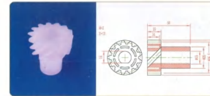
品名: 16齿40直齿轮 规格: M2.5×16Z 材质: PP 编号: CT-ZCL-066
