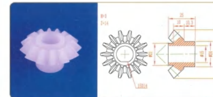
品名: 14齿伞齿轮 规格: M3×14Z×25L 材质: PVDF 编号: CT-SCL-008
