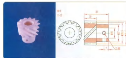
品名: 12齿螺旋齿轮 规格: M2×12Z×38L 材质: PE 编号: CT-LXCL-047
