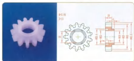
品名: 13齿40直齿轮 规格: M3×13Z 材质: PVDF 编号: CT-ZCL-063
