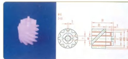
品名: 10齿螺旋齿轮 规格: M2×10Z×35L 材质: PVDF 编号: CT-LXCL-021
