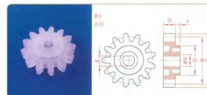
品名: 13齿40直齿轮 规格: M3×13Z 材质: PP 编号: CT-ZCL-057
