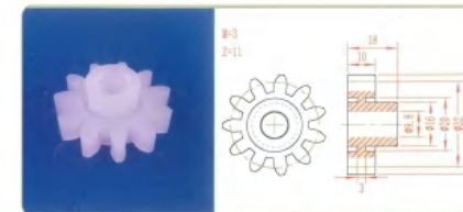
品名: 11齿32直齿轮 规格: M3×11Z 材质: PVDF 编号: CT-ZCL-032
