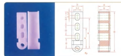
品名: 65插件 材质: PF
