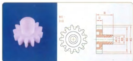
品名: 13齿40直齿轮 规格: M3×13Z 材质: PP 编号: CT-ZCL-061
