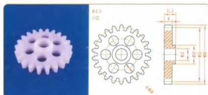
品名: 22齿55直齿轮 规格: M2.5×22Z 材质: PP 编号: CT-ZCL-105
