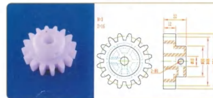
品名: 16齿48直齿轮 规格: M3×16Z 材质: PP 编号: CT-ZCL-080
