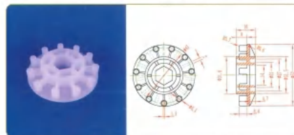
品名: 11齿钉齿轮 规格: 11Z×Φ52×16L 材质: PVDF 编号: CT-DCL-016
