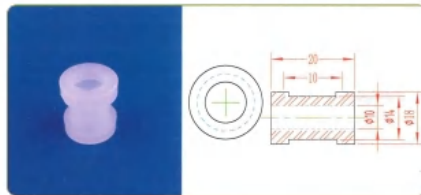
品名: Φ10轴套 规格: Φ10×20L 材质: PVDF 编号: CT-ZT-008
