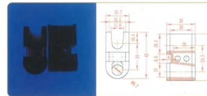
品名: 24插件 材质: PE
