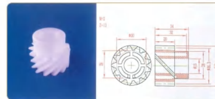
品名: 13齿螺旋齿轮 规格: M3×13Z 材质: UPE 编号: CT-ZCL-061
