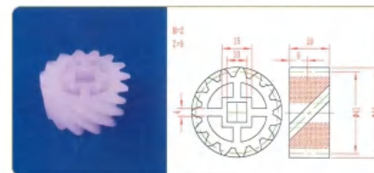
品名: 16齿40直齿轮 规格: M2.5×16Z 材质: PP 编号: CT-ZCL-067
