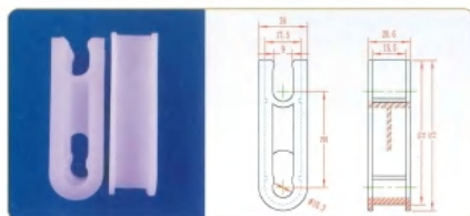
品名: 50插件 材质: PP
