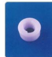
品名: Φ12.5固定套 规格: Φ12.5×14L 材质: PP 编号: CT-SJT-030
