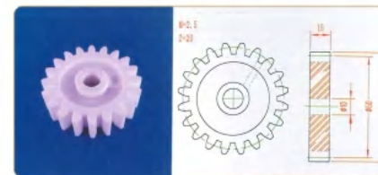
品名: 20齿50直齿轮 规格: M2.5×20Z 材质: PP 编号: CT-ZCL-099
