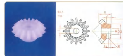
品名: 16齿伞齿轮 材质: UPE
