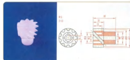
品名: 10齿螺旋齿轮 规格: M2×10Z×38L 材质: PP 编号: CT-LXCL-025
