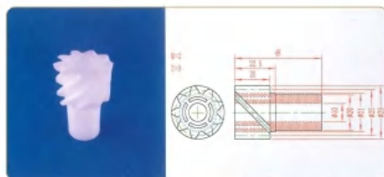
品名: 9齿螺旋齿轮 规格: M2×9Z×48L 材质: UPE 编号: CT-LXCL-011
