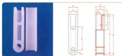
品名: 50插件 材质: PVDF
