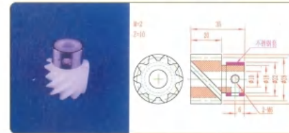
品名: 10齿螺旋齿轮 规格: M2×10Z×35L 材质: UPE 编号: CT-LXCL-024
