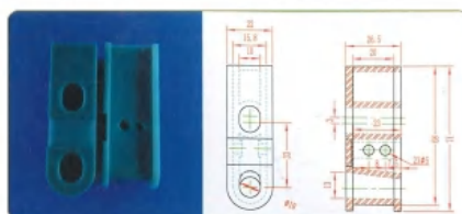
品名: 33插件 材质: PE
