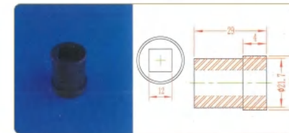
品名: 方12轴套 规格: 方孔12×29L 材质: 铁氟龙 编号: CT-ZT-016
