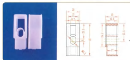
品名: 45上插件 材质: HCPP/PVDF
