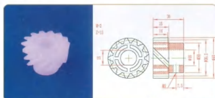
品名: 13齿螺旋齿轮 规格: M2×13Z×30L 材质: PVDF 编号: CT-LXCL-053
