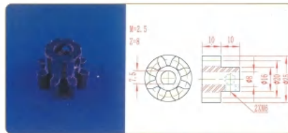
品名: 8齿20直齿轮 材质: PVC
