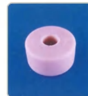
品名: \Phi 32 滚轮片 规格: \Phi 32 \times \Phi 9.8 \times 17L \times 17W 平面 材质: 孟山都 编号: CT-LP-234
