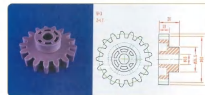
品名: 17齿50直齿轮 规格: M3×17Z 材质: PP 编号: CT-ZCL-095
