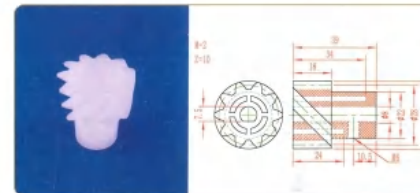
品名: 10齿螺旋齿轮 规格: M2×10Z×39L 材质: PVDF 编号: CT-LXCL-028
