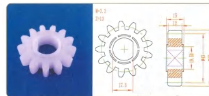
品名: 13齿43直齿轮 规格: M3.25×13Z 材质: PP 编号: CT-ZCL-078
