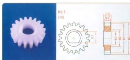
品名: 18齿45直齿轮 规格: M2.5×18Z 材质: PP 编号: CT-ZCL-081
