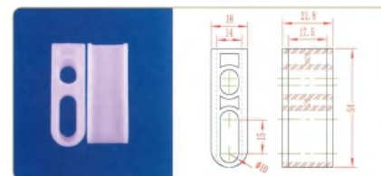
品名: 30插件 材质: PE
