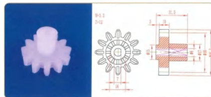
品名: 12齿40直齿轮 规格: M3.3×12Z 材质: PVDF 编号: CT-ZCL-050
