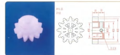
品名: 12齿40直齿轮 规格: M3.25×12Z 材质: PVDF 编号: CT-ZCL-054
