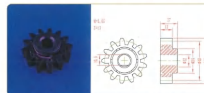
品名: 13齿40直齿轮 规格: M3.05×13Z 材质: PPF 编号: CT-ZCL-055
