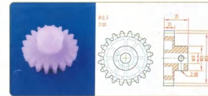
品名: 20齿50直齿轮 规格: M2.5×20Z 材质: PVDF 编号: CT-ZCL-100
