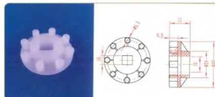
品名: 8齿钉齿轮 规格: 8Z×Φ40×13L 材质: PVDF 编号: CT-DCL-005
