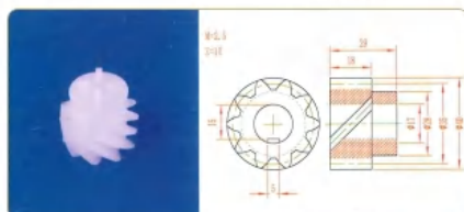
品名: 10齿螺旋齿轮 规格: M2.5×10Z×35L 材质: PVDF 编号: CT-LXCL-035
