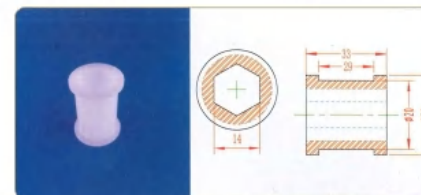
品名: 六角14轴套 规格: 六角14×33L 材质: PE 编号: CT-ZT-019
