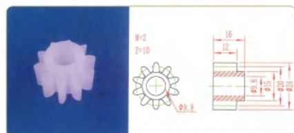
品名: 10齿20直齿轮 材质: PVDF
