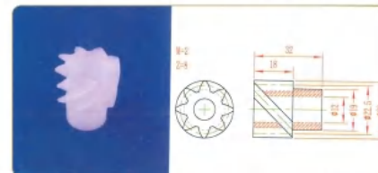
品名: 8齿螺旋齿轮 规格: M2×8Z×32L 材质: UPE 编号: CT-LXCL-005
