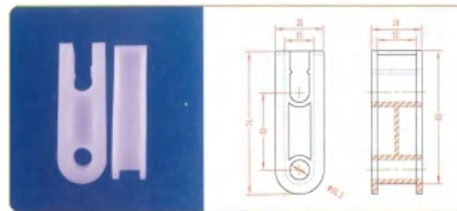
品名: 40插件 材质: PE
