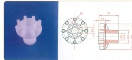
品名: 8齿钉齿轮 规格: 8Z×Φ31×33L 材质: PP 编号: CT-DCL-002
