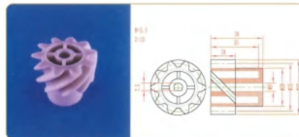
品名: 10齿螺旋齿轮 规格: M2.5×10Z×38L 材质: PP 编号: CT-LXCL-074
