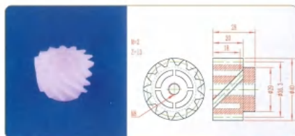
品名: 13齿螺旋齿轮 规格: M2×13Z×28L 材质: PVDF 编号: CT-LXCL-051
