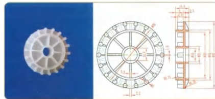
品名: 18齿钉齿轮 规格: 18Z×Φ81×15.9L 材质: PP 编号: CT-DCL-020
