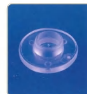
品名: \Phi 30 滚轮片 规格: \Phi 30 \times \Phi 11 \times 13L \times 3.5W 平面 材质: PVC 编号: CT-LP-232
