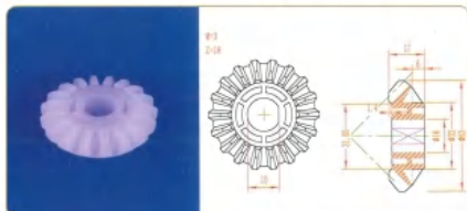
品名: 18齿伞齿轮 规格: M3×18Z×17I 材质: PVDF 编号: CT-SCL-036
