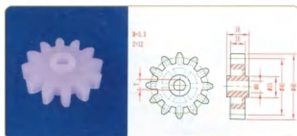
品名: 12齿40直齿轮 规格: M3.3×12Z 材质: PVDF 编号: CT-ZCL-049
