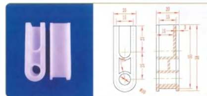
品名: 25插件 材质: PE/PVDF
