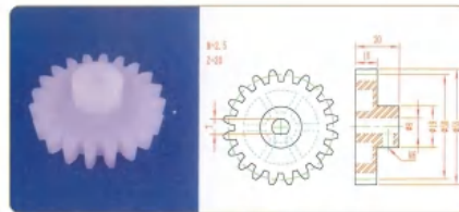
品名: 20齿50直齿轮 规格: M2.5×20Z 材质: PVDF 编号: CT-ZCL-102
