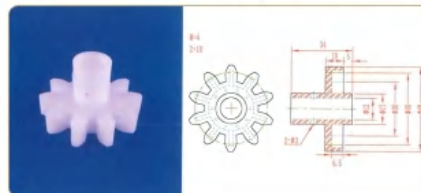
品名: 10齿40直齿轮 规格: M4×10Z 材质: PP 编号: CT-ZCL-046
