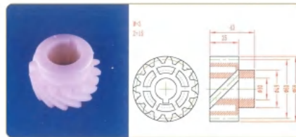
品名: 15齿螺旋齿轮 规格: M3×15Z×43L 材质: UPE 编号: CT-LXCL-072
