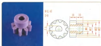
品名: 9齿22直齿轮 规格: M2.45×9Z 材质: PVC 编号: CT-ZCL-107
