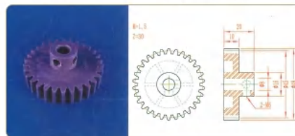
品名: 30齿45直齿轮 规格: M1.5×30Z 材质: PP 编号: CT-ZCL-086
