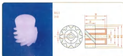
品名: 10齿螺旋齿轮 规格: M2.5×10Z×38L 材质: PVDF 编号: CT-LXCL-037
