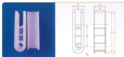
品名: 40插件 材质: PVDF
