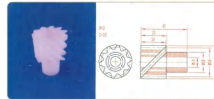
品名: 10齿螺旋齿轮 规格: M2×10Z×45L 材质: PVDF 编号: CT-LXCL-030
