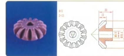
品名: 13齿伞齿轮 规格: M3×13Z×20L 材质: PEEK 编号: CT-SCL-004
