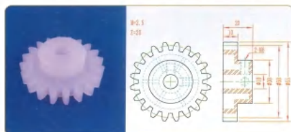
品名: 20齿50直齿轮 规格: M2.5×20Z 材质: PVDF 编号: CT-ZCL-103
