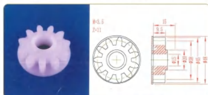
品名: 11齿38直齿轮 规格: M3.5×11Z 材质: PP 编号: CT-ZCL-045
