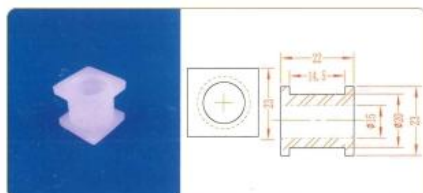
品名: \Phi 15 轴套 规格: \Phi 15 \times 22L 材质: PVDF 编号: CT-ZT-025
