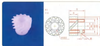
品名: 13齿螺旋齿轮 规格: M2×13Z×33L 材质: PVDF 编号: CT-LXCL-058
