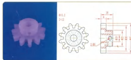
品名: 12齿40直齿轮 规格: M3.2×12Z 材质: PVDF 编号: CT-ZCL-048
