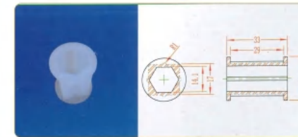
品名: 六角14轴套 规格: 六角14×33L 材质: PE 编号: CT-ZT-020
