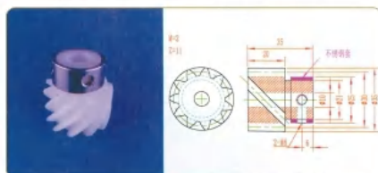
品名: 11齿螺旋齿轮 规格: M2×11Z×35L 材质: UPE 编号: CT-LXCL-039
