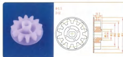
品名: 12齿42直齿轮 规格: M3.5×12Z 材质: PP 编号: CT-ZCL-073
