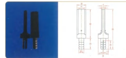
品名: 插板 材质: PP
