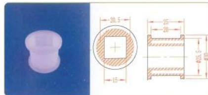
品名: 方孔15轴套 规格: 方孔15 \times 25L 材质: PE 编号: CT-ZT-022
