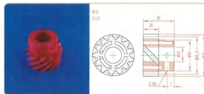
品名: 13齿螺旋齿轮 规格: M2×13Z×34L 材质: PVDF 编号: CT-LXCL-060
