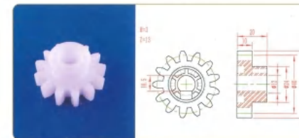
品名: 13齿40直齿轮 规格: M3×13Z 材质: PP 编号: CT-ZCL-058
