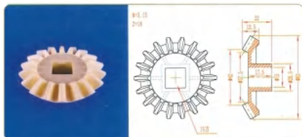
品名: 18齿伞齿轮 规格: M3.15×18Z×22L 材质: PE 编号: CT-SCL-038
