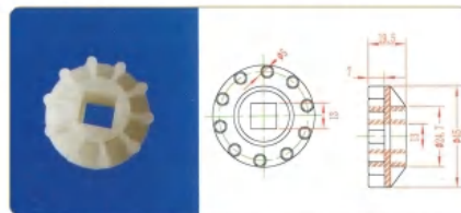
品名: 10齿钉齿轮 规格: 10Z×Φ45×19.5L 材质: PVDF 编号: CT-DCL-018
