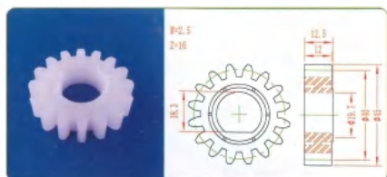
品名: 16齿40直齿轮 规格: M2.5×16Z 材质: PP 编号: CT-ZCL-069
