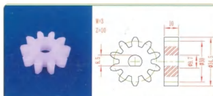
品名: 10齿30直齿轮 规格: Φ10×78H 材质: PVDF 编号: CT-CX-135
