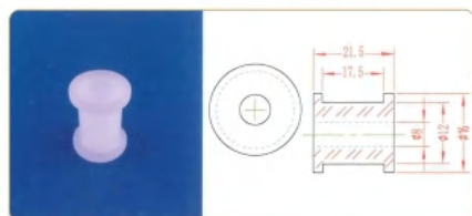
品名: Φ8轴套 规格: Φ8×21.5L 材质: PE 编号: CT-ZT-003
