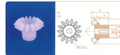
品名: 14齿伞齿轮 规格: M3×14Z×33L 材质: PVDF 编号: CT-SCL-010
