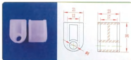
品名: 30下插件 材质: PVDF
