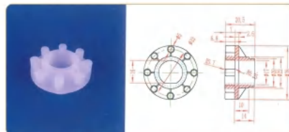
品名: 8齿钉齿轮 规格: 8Z×Φ38×20.5L 材质: PVDF 编号: CT-DCL-003
