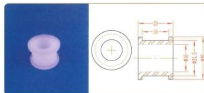
品名: \Phi 16 轴套 规格: \Phi 16 \times 20L 材质: PVDF 编号: CT-ZT-028
