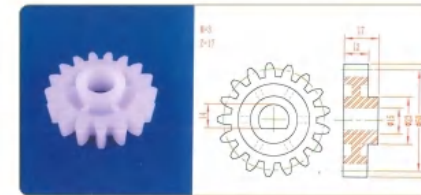
品名: 17齿50直齿轮 规格: M3×17Z 材质: PP 编号: CT-ZCL-096
