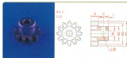
品名: 12齿30直齿轮 规格: M2.5×12Z 材质: PVC 编号: CT-ZCL-028
