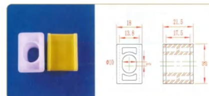
品名: 30上插件 材质: PE 规格: Φ10×28H 编号: CT-CX-005
