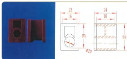
品名: 下插件 材质: 尼龙
