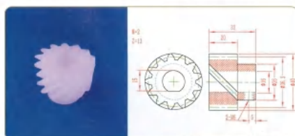
品名: 13齿螺旋齿轮 规格: M2×13Z×33L 材质: PVDF 编号: CT-LXCL-059
