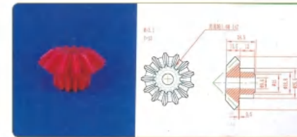
品名: 一体组合齿轮 规格: 13Z伞+14Z直×24.5L 材质: PVDF 编号: CT-ZHCL-008
