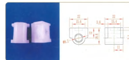
品名: 下插件 材质: PP/PVDF
