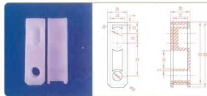
品名: 32插件 材质: PVDE
