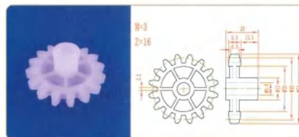
品名: 16齿48直齿轮 规格: M3×16Z 材质: PVDF 编号: CT-ZCL-088
