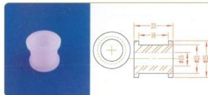
品名: \Phi 15 轴套 规格: \Phi 15 \times 23L 材质: PVDF 编号: CT-ZT-026
