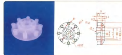
品名: 8齿钉齿轮 规格: 8Z×Φ40×15L 材质: PVDF 编号: CT-DCL-006
