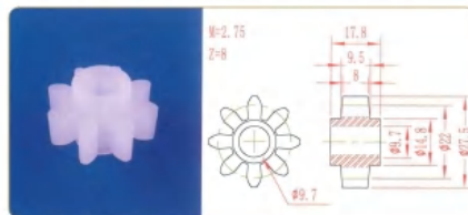
品名: 11齿22直齿轮 材质: PP/PEEK
