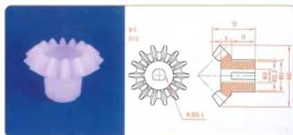
品名: 14齿伞齿轮 材质: PVDF
