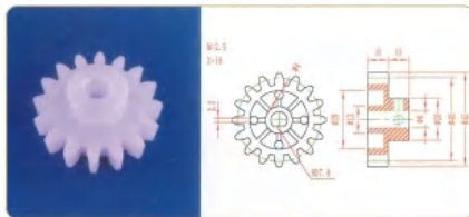
品名: 16齿40直齿轮 规格: M2.5×16Z 材质: PE 编号: CT-ZCL-064
