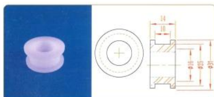
品名: \Phi 16 轴套 规格: \Phi 16 \times 14L 材质: UPE 编号: CT-ZT-027
