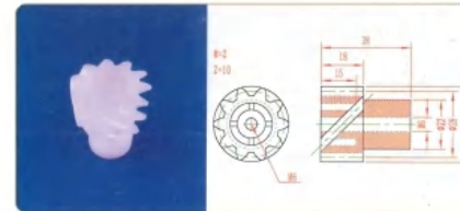
品名: 10齿螺旋齿轮 规格: M2×10Z×38L 材质: PP 编号: CT-LXCL-026
