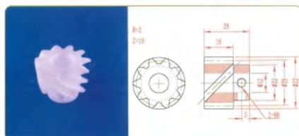
品名: 10齿螺旋齿轮 规格: M2×10Z×28L 材质: UPE 编号: CT-LXCL-015
