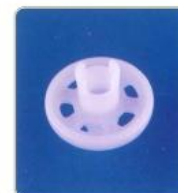
品名: Φ30滚轮片 规格: Φ30×Φ8×20L×5W平面 材质: PP 编号: CT-LP-022
