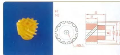
品名: 12齿螺旋齿轮 规格: M2×12Z×32L 材质: PE 编号: CT-LXCL-041
