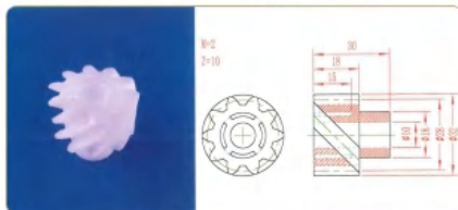
品名: 10齿螺旋齿轮 规格: M2×10Z×30L 材质: UPE 编号: CT-LXCL-016
