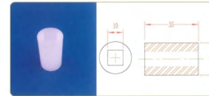
品名: 方10轴套 规格: 方孔10×35L 材质: PVDF 编号: CT-ZT-014
