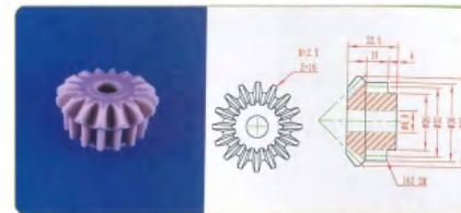
品名: 一体组合齿轮 规格: 16Z伞+16Z直×22.5L 材质: 德灰PP 编号: CT-ZHCL-009
