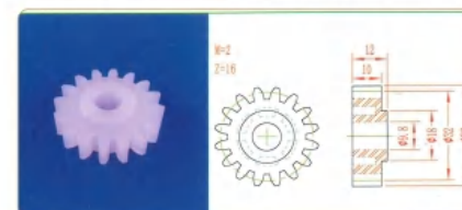
品名: 16齿32直齿轮 规格: M2×16Z 材质: PVDF 编号: CT-ZCL-039
