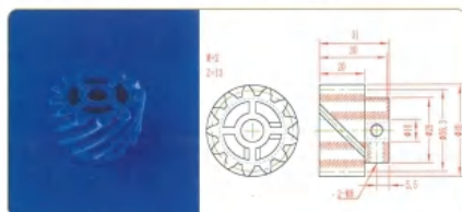
品名: 13齿螺旋齿轮 规格: M2×13Z×31L 材质: PF 编号: CT-LXCL-055
