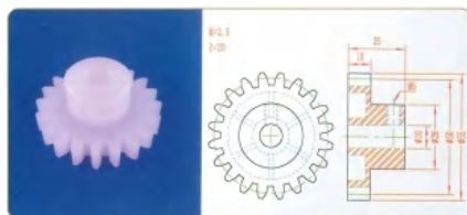
品名: 20齿50直齿轮 规格: M2.5×20Z 材质: PVDF 编号: CT-ZCL-101
