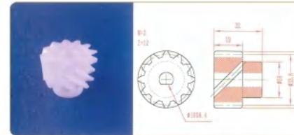
品名: 12齿螺旋齿轮 规格: M2×12Z×32L 材质: PE 编号: CT-LXCL-042
