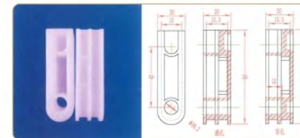
品名: 43插件 材质: PE
