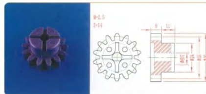
品名: 14齿35直齿轮 规格: M2.5×14Z 材质: PVC 编号: CT-ZCL-044
