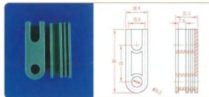
品名: 33插件 材质: PE
