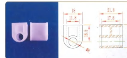
品名: 30下插件 材质: UPE 规格: Φ8×22.5H 编号: CT-CX-008
