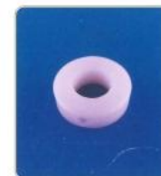
品名: Φ15固定套 规格: Φ15×10L 材质: PP 编号: CT-SJT-032
