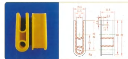
品名: 25插件 材质: PE
