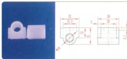
品名: 下插件 材质: PVDF
