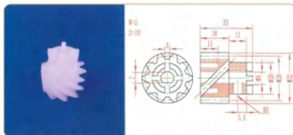
品名: 10齿螺旋齿轮 规格: M2×10Z×33L 材质: PVDF 编号: CT-LXCL-020
