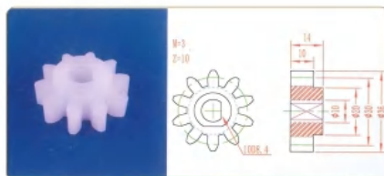
品名: 10齿30直齿轮 规格: M3×10Z 材质: PP 编号: CT-ZCL-021
