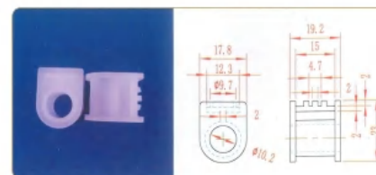
品名: 25上插件 材质: PVDF 规格: Φ10×23H 编号: CT-CX-001
