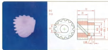
品名: 13齿螺旋齿轮 规格: M2×13Z×30L 材质: PE 编号: CT-LXCL-052
