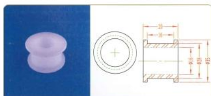
品名: \Phi 16 轴套 规格: \Phi 16 \times 20L 材质: UPE 编号: CT-ZT-029
