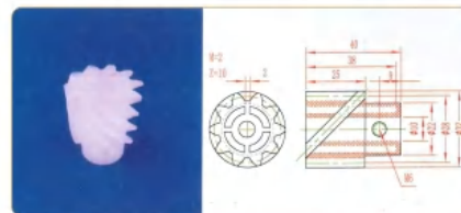
品名: 10齿螺旋齿轮 规格: M2×10Z×40L 材质: PVDF 编号: CT-LXCL-029
