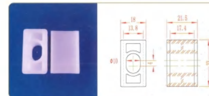
品名: 30上插件 材质: PE 规格: Φ10×33H 编号: CT-CX-006
