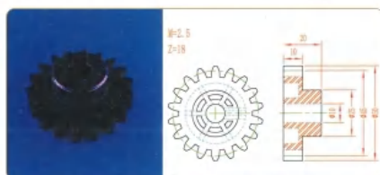
品名: 18齿45直齿轮 规格: M2.5×18Z 材质: PVDF 编号: CT-ZCL-085
