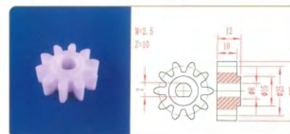
品名: 10齿25直齿轮 材质: PP
