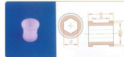
品名: 六角17轴套 规格: 六角17 \times 33L 材质: PVDF 编号: CT-ZT-034
