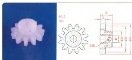
品名: 12齿40直齿轮 规格: M3.2×12Z 材质: PVDF 编号: CT-ZCL-047
