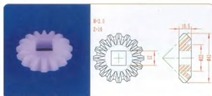
品名: 16齿伞齿轮 材质: PVDF
