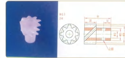
品名: 8齿螺旋齿轮 规格: M2.5×8Z×44L 材质: UPE 编号: CT-LXCL-002
