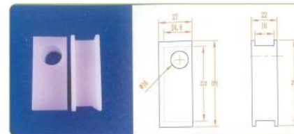
品名: \Phi 16 轴套 规格: \Phi 16 \times 58L 材质: UPE 编号: CT-ZT-031
