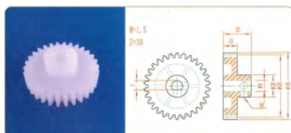
品名: 30齿45直齿轮 规格: M1.5×30Z 材质: PP 编号: CT-ZCL-087
