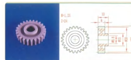
品名: 24齿30直齿轮 规格: M1.25×24Z 材质: PP 编号: CT-ZCL-031
