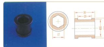
品名: 六角17轴套 规格: 六角17 \times 30L 材质: 铁氟龙 编号: CT-ZT-033
