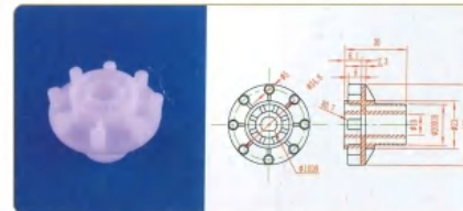
品名: 8齿钉齿轮 规格: 8Z×Φ40×30L 材质: PP 编号: CT-DCL-010
