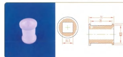
品名: 方10轴套 规格: 方孔10×31L 材质: UPE 编号: CT-ZT-015
