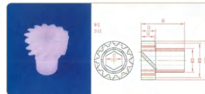
品名: 16齿40直齿轮 规格: M2.5×16Z 材质: PP 编号: CT-ZCL-065
