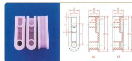
品名: 43插件 材质: PVDF
