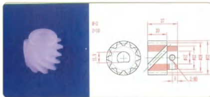
品名: 10齿螺旋齿轮 规格: M2×10Z×27L 材质: PVDF 编号: CT-LXCL-012
