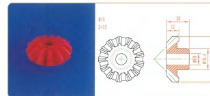
品名: 13齿伞齿轮 规格: M3×13Z×20L 材质: PVDF 编号: CT-SCL-003
