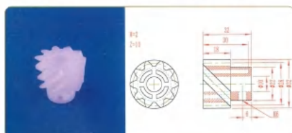
品名: 10齿螺旋齿轮 规格: M2×10Z×321 材质: PVDF 编号: CT-LXCL-017
