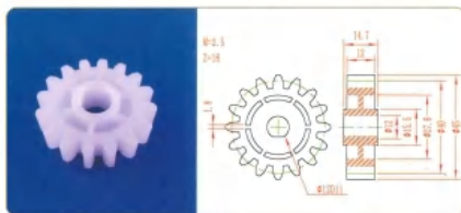
品名: 16齿40直齿轮 规格: M2.5×16Z 材质: PP 编号: CT-ZCL-068
