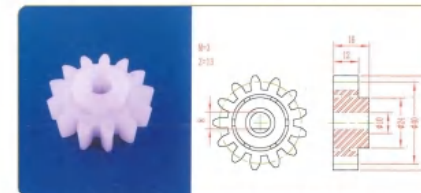
品名: 13齿40直齿轮 规格: M3×13Z 材质: PP 编号: CT-ZCL-056
