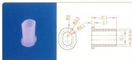
品名: \Phi 15 轴套 规格: \Phi 15 \times 27.3L 材质: UPE 编号: CT-ZT-021
