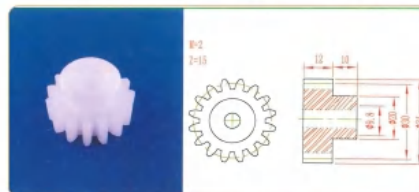
品名: 15齿30直齿轮 规格: M2×15Z 材质: PP 编号: CT-ZCL-030
