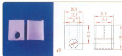
品名: 40下插件 材质: PVDF
