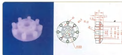
品名: 8齿钉齿轮 规格: 8Z×Φ40×15L 材质: PVDF 编号: CT-DCL-007
