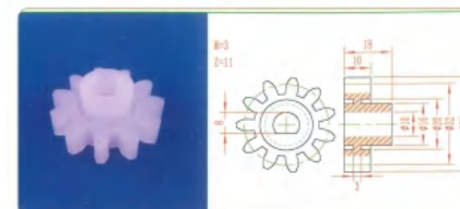
品名: M3×11Z 规格: PVDF 材质: PVDF 编号: CT-ZCL-033
