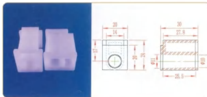
品名: 下插件 材质: PE
