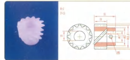
品名: 12齿螺旋齿轮 规格: M2×12Z×32L 材质: PE 编号: CT-LXCL-044
