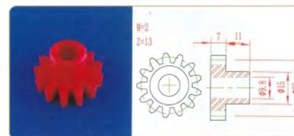
品名: 13齿26直齿轮 材质: PVDF
