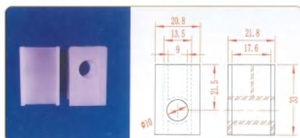
品名: 40上插件 材质: PVDF
