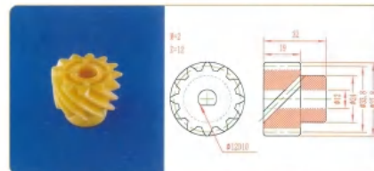
品名: 12齿螺旋齿轮 规格: M2×12Z×32L 材质: PE 编号: CT-LXCL-043
