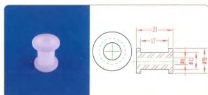
品名: Φ8轴套 规格: Φ8×21L 材质: UPE 编号: CT-ZT-005
