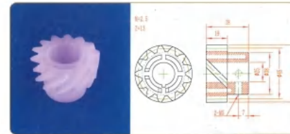
品名: 13齿螺旋齿轮 规格: M2.5×13Z×38L 材质: PVDF 编号: CT-LXCL-048
