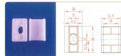
品名: 30上插件 材质: PE 规格: Φ8×30H 编号: CT-CX-004
