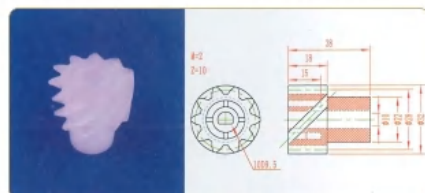
品名: 10齿螺旋齿轮 规格: M2×10Z×38L 材质: PVDF 编号: CT-1XCL-075
