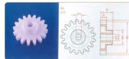
品名: 17齿50直齿轮 规格: M3×17Z 材质: PP 编号: CT-ZCL-091
