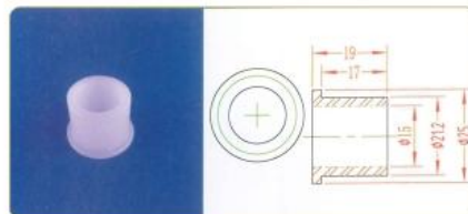
品名: \Phi 15 轴套 规格: \Phi 15 \times 19L 材质: UPE 编号: CT-ZT-024
