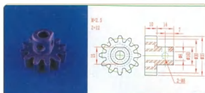
品名: 12齿30直齿轮 规格: M2.5×12Z 材质: PVC 编号: CT-ZCL-029
