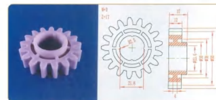
品名: 17齿50直齿轮 规格: M3×17Z 材质: PP 编号: CT-ZCL-093
