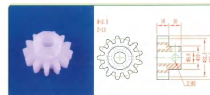
品名: 13齿32直齿轮 规格: M2.5×13Z 材质: PP 编号: CT-ZCL-035
