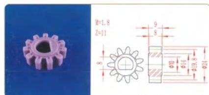
品名: 11齿22直齿轮 材质: PVDF/PEEK
