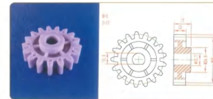
品名: 17齿50直齿轮 规格: M3×17Z 材质: PP 编号: CT-ZCL-092
