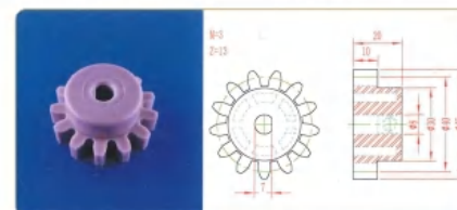
品名: 13齿40直齿轮 规格: M3×13Z 材质: PP 编号: CT-ZCL-059
