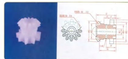
品名: 一体组合齿轮 规格: 12Z伞+10Z直×41 材质: PP 编号: CT-ZHCL-007
