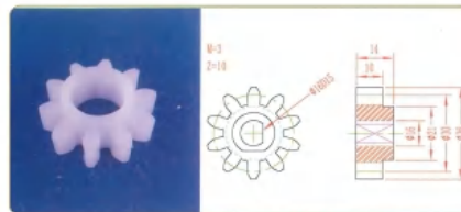
品名: 10齿30直齿轮 规格: M3×10Z 材质: PP 编号: CT-ZCL-022
