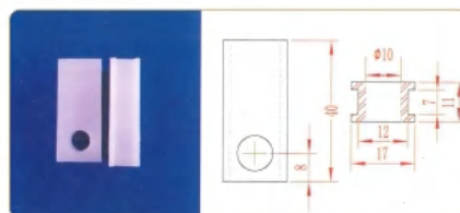
品名: 45下插件 材质: PP
