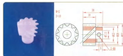
品名: 10齿螺旋齿轮 规格: M2×10Z×38L 材质: UPF 编号: CT-LXCL-027
