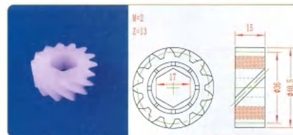
品名: 13齿螺旋齿轮 规格: M2×13Z×15L 材质: PVDF 编号: CT-LXCL-049
