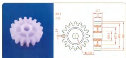
品名: 16齿40直齿轮 规格: M2.5×16Z 材质: PP 编号: CT-ZCL-067
