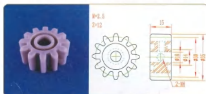
品名: 12齿30直齿轮 规格: M2.5×12Z 材质: PP 编号: CT-ZCL-109
