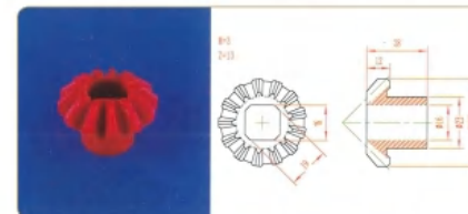
品名: 13齿伞齿轮 规格: M3×13Z×28L 材质: PVDF 编号: CT-SCL-005
