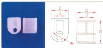
品名: 30下插件 材质: PVDF
