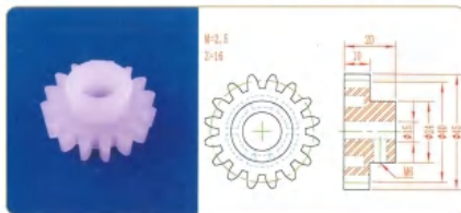
品名: 16齿40直齿轮 规格: M2.5×16Z 材质: PVDF 编号: CT-ZCL-070
