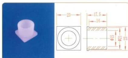
品名: \Phi 15 轴套 规格: \Phi 15 \times 17.5L 材质: PVDF 编号: CT-ZT-023
