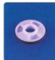
品名: \Phi 45 滚轮片 规格: \Phi 45 \times \Phi 15 \times 10L \times 6W 弧面 材质: PP+EPDM 编号: CT-LP-215
