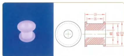
品名: Φ8轴套 规格: Φ8×19L 材质: UPE 编号: CT-ZT-001
