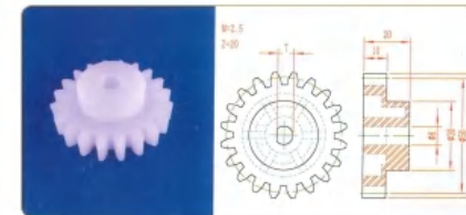
品名: 20齿50直齿轮 规格: M2.5×20Z 材质: PP 编号: CT-ZCL-098
