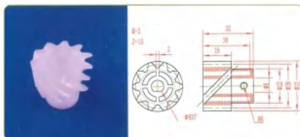
品名: 10齿螺旋齿轮 规格: M2×10Z×32L 材质: PVDF 编号: CT-LXCL-018
