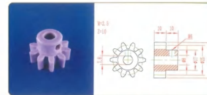
品名: 10齿25直齿轮 材质: PP/PVC/PVDF
