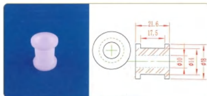
品名: Φ10轴套 规格: Φ10×21.5L 材质: PE 编号: CT-ZT-010
