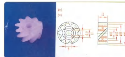
品名: 9齿螺旋齿轮 规格: M2×9Z×12L 材质: PVDF 编号: CT-LXCL-007
