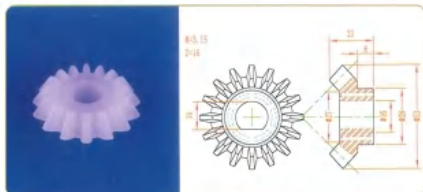
品名: 16齿伞齿轮 规格: M3.15×16Z×23L 材质: PVDF 编号: CT-SCL-034
