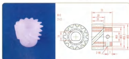
品名: 13齿螺旋齿轮 规格: M2×13Z×33L 材质: PVDF 编号: CT-LXCL-057
