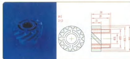
品名: 13齿螺旋齿轮 规格: M2×13Z×30L 材质: 尼龙 编号: CT-LXCL-054
