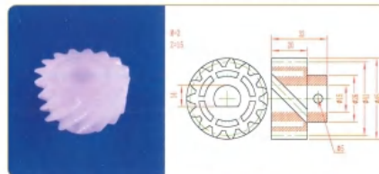
品名: 15齿螺旋齿轮 规格: M2×15Z×31L 材质: PE 编号: CT-LXCL-076
