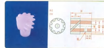
品名: 9齿螺旋齿轮 规格: M2×9Z×38L 材质: UPE 编号: CT-LXCL-010
