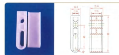
品名: 40插件 材质: PE
