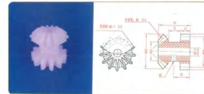
品名: 分体组合齿轮 规格: 13Z伞+12Z直×40L 材质: PVDF 编号: CT-ZHCL-006
