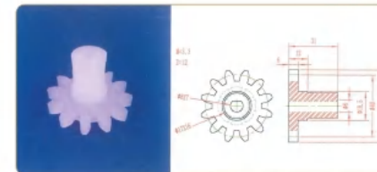
品名: 12齿40直齿轮 规格: M3.3×12Z 材质: PVDF 编号: CT-ZCL-052
