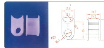
品名: 25下插件 材质: PVDF 规格: Φ10×30H 编号: CT-CX-002
