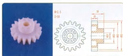
品名: 18齿45直齿轮 规格: M2.5×18Z 材质: PP 编号: CT-ZCL-083
