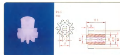
品名: 10齿25直齿轮 材质: PVDF
