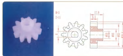
品名: 11齿33直齿轮 规格: M3×11Z 材质: PVDF 编号: CT-ZCL-042
