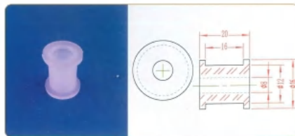
品名: Φ8轴套 规格: Φ8×20L 材质: PVDF 编号: CT-ZT-002
