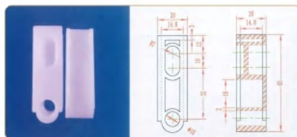
品名: 32插件 材质: PE
