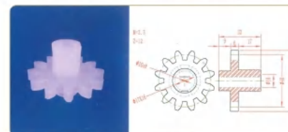
品名: 12齿40直齿轮 规格: M3.3×12Z 材质: PVDF 编号: CT-ZCL-053
