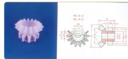
品名: 分体组合齿轮 规格: 14Z伞+10Z直×32L 材质: PVDF 编号: CT-ZHCL-001
