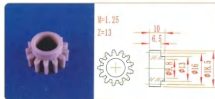
品名: 13齿16直齿轮 规格: M1.25×13Z 材质: PP 编号: CT-ZCL-110
