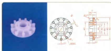
品名: 11齿钉齿轮 规格: 11Z×Φ52×16L 材质: PVDF 编号: CT-DCL-015
