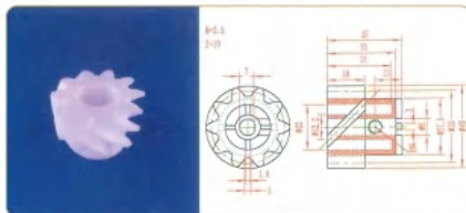
品名: 10齿螺旋齿轮 规格: M2.5×10Z×29L 材质: PE 编号: CT-LXCL-034
