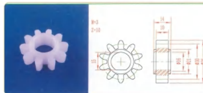
品名: 10齿30直齿轮 规格: M3×10Z 材质: PP 编号: CT-ZCL-024
