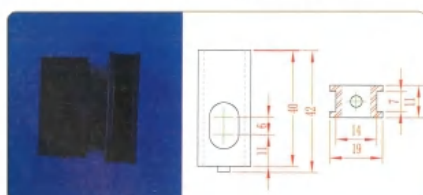
品名: 45上插件 材质: MC
