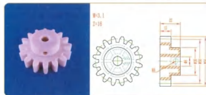
品名: 16齿50直齿轮 规格: M3.1×16Z 材质: PP 编号: CT-ZCL-090
