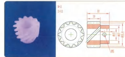
品名: 12齿螺旋齿轮 规格: M2×12Z×32L 材质: PE 编号: CT-LXCL-046
