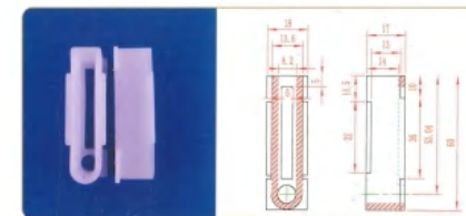
品名: 38插件 材质: PVDF
