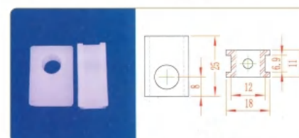
品名: 下插件 材质: PVDF
