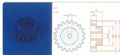
品名: 20齿40直齿轮 规格: M2×20Z 材质: PP 编号: CT-ZCL-071
