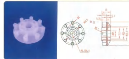
品名: 8齿钉齿轮 规格: 8Z×Φ39.5×15L 材质: PVDF 编号: CT-DCL-004
