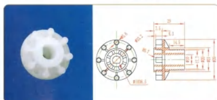
品名: 8齿钉齿轮 规格: 8Z×Φ39×15L 材质: PVDF 编号: CT-DCL-017
