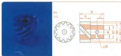
品名: 11齿螺旋齿轮 规格: M2×11Z×40L 材质: 尼龙 编号: CT-LXCL-040
