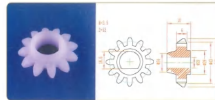
品名: 12齿42直齿轮 规格: M3.5×12Z 材质: PP 编号: CT-ZCL-072
