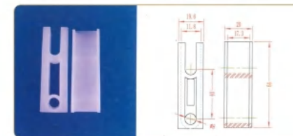
品名: 40插件 材质: PVDF
