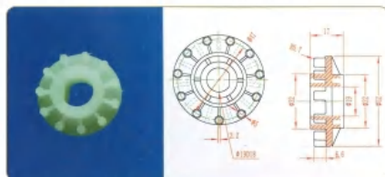
品名: 11齿钉齿轮 规格: 11Z×Φ52×17L 材质: PVDF 编号: CT-DCL-019
