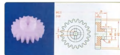
品名: 20齿50直齿轮 规格: M2.5×20Z 材质: PP 编号: CT-ZCL-097
