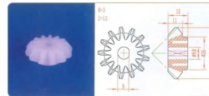
品名: 13齿伞齿轮 规格: M3×13Z×15L 材质: PVDF 编号: CT-SCI-001
