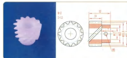
品名: 12齿螺旋齿轮 规格: M2×12Z×32L 材质: PE 编号: CT-LXCL-045
