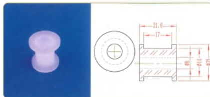
品名: Φ8轴套 规格: Φ8×21.5L 材质: PVDF 编号: CT-ZT-004
