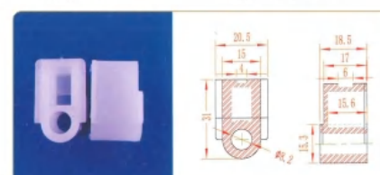
品名: 下插件 材质: HCPP/PVDF
