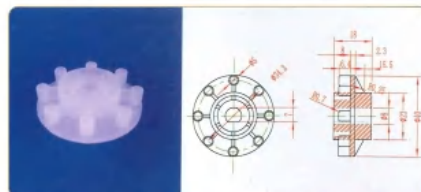
品名: 8齿钉齿轮 规格: 8Z×Φ40×18L 材质: PVDF 编号: CT-DCL-009
