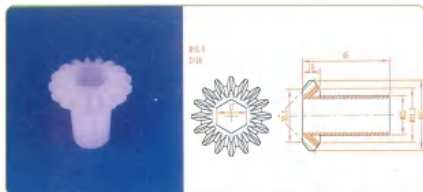
品名: 16齿伞齿轮 规格: M2.5×16Z×45I 材质: PVDF 编号: CT-SCL-032
