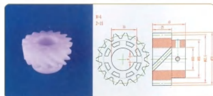
品名: 15齿螺旋齿轮 规格: M4×15Z×43L 材质: UPE 编号: CT-LXCL-073
