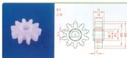
品名: 10齿30直齿轮 规格: M3×10Z 材质: PP 编号: CT-ZCL-023
