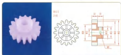
品名: 16齿40直齿轮 规格: M2.5×16Z 材质: PP 编号: CT-ZCL-065
