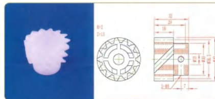
品名: 13齿螺旋齿轮 规格: M2×13Z×32L 材质: PVDF 编号: CT-LXCL-056
