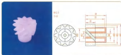
品名: 10齿螺旋齿轮 规格: M2.5×10Z×38L 材质: PVDF 编号: CT-LXCL-036
