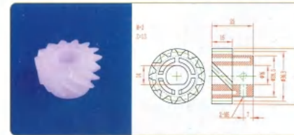
品名: 13齿螺旋齿轮 规格: M2×13Z×25L 材质: PVDF 编号: CT-LXCL-050
