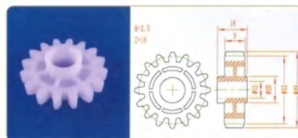
品名: 16齿43直齿轮 规格: M2.5×16Z 材质: PP 编号: CT-ZCL-079
