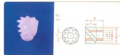
品名: 8齿螺旋齿轮 规格: M2×8Z×28L 材质: UPE 编号: CT-LXCL-003
