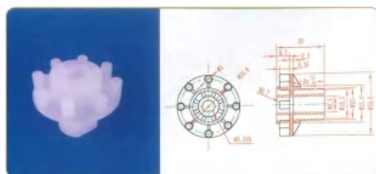
品名: 8齿钉齿轮 规格: 8Z×Φ40×30L 材质: PVDF 编号: CT-DC1-011
