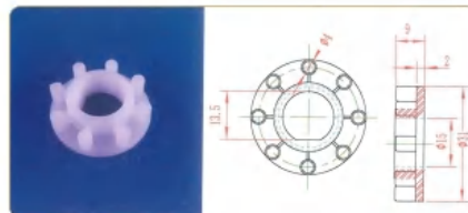
品名: 8齿钉齿轮 规格: 8Z×Φ31×9L 材质: PP 编号: CT-DCL-001
