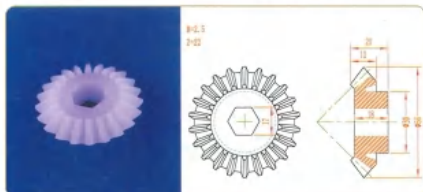
品名: 22齿伞齿轮 规格: M3×22Z×20L 材质: PVDF 编号: CT-SCL-040
