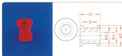
品名: Φ10.5轴套 规格: Φ10.5×26L 材质: UPE 编号: CT-ZT-006
