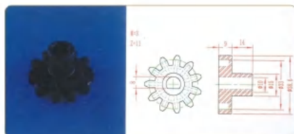
品名: 11齿33直齿轮 规格: M3×11Z 材质: PVDF 编号: CT-ZCL-041
