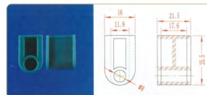
品名: 30下插件 材质: PE 规格: Φ8×25.5H 编号: CT-CX-009
