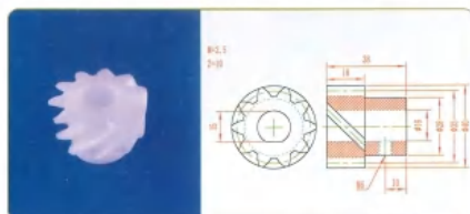
品名: 10齿螺旋齿轮 规格: M2.5×10Z×29L 材质: PE 编号: CT-LXCL-033
