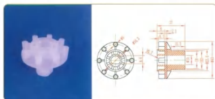
品名: 8齿钉齿轮 规格: 8Z×Φ40×31L 材质: PVDF 编号: CT-DCL-013
