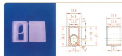
品名: 30上插件 材质: HCPP 规格: Φ8×26.2H 编号: CT-CX-003
