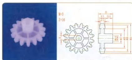
品名: 16齿48直齿轮 规格: M3×16Z 材质: PVDF 编号: CT-ZCL-089
