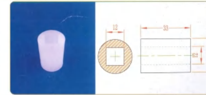
品名: 方12轴套 规格: 方孔12×33L 材质: PVDF 编号: CT-ZT-018
