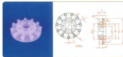
品名: 11齿钉齿轮 规格: 11Z×Φ52×16L 材质: PVDF 编号: CT-DCL-014
