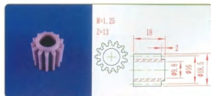
品名: 13齿16直齿轮 材质: PP/PVDF
