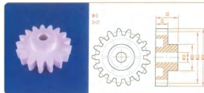
品名: 17齿53直齿轮 规格: M3×17Z 材质: PP 编号: CT-ZCL-104
