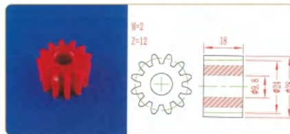
品名: 12齿26直齿轮 材质: PVDF
