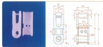
品名: 33插件 材质: PVDF
