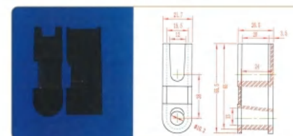
品名: 38插件 材质: PE
