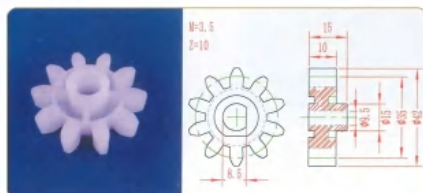
品名: 10齿35直齿轮 规格: M3.5×10Z 材质: PP 编号: CT-ZCL-043
