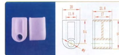
品名: 30下插件 材质: PE 规格: Φ8×33H 编号: CT-CX-010
