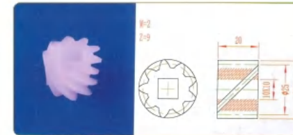
品名: 9齿螺旋齿轮 规格: M2×9Z×20L 材质: PVDF 编号: CT-LXCL-008
