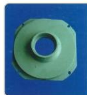
品名: 离台防水套固定座 规格: ST-38 材质: A3钢 编号: CT-jGj-027
