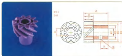
品名: 10齿螺旋齿轮 规格: M2.5×10Z×45L 材质: PVC 编号: CT-LXCL-038
