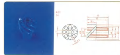
品名: 8齿螺旋齿轮 规格: M2.5×8Z×44L 材质: UPE 编号: GYK-LXCL-001
