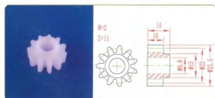
品名: 11齿22直齿轮 材质: PP
