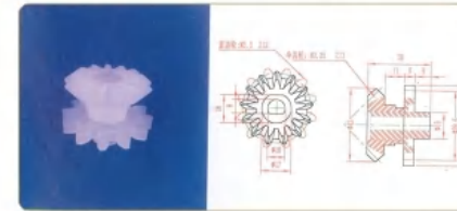
品名: 分体组合齿轮 规格: 13Z伞+12Z直×36L 材质: PVDF 编号: CT-ZHCL-004
