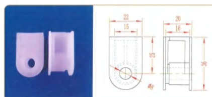
品名: 50下插件 材质: PE
