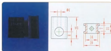
品名: 30下插件 材质: MC
