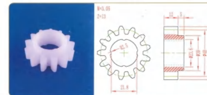
品名: 13齿40直齿轮 规格: M3×13Z 材质: PP 编号: CT-ZCL-060
