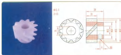
品名: 10齿螺旋齿轮 规格: M2.5×10Z×29L 材质: PE 编号: CT-LXCL-032
