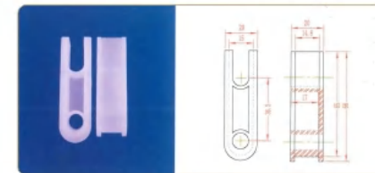
品名: 36.5插件 材质: PVDF
