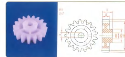
品名: 17齿50直齿轮 规格: M3×17Z 材质: PP 编号: CT-ZCL-094
