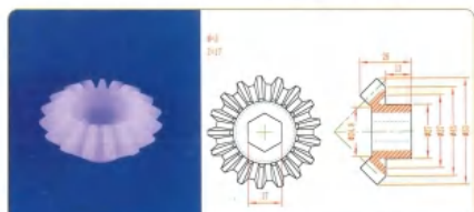
品名: 17齿伞齿轮 规格: M3×17Z×26L 材质: PVDF 编号: CT-SCL-035
