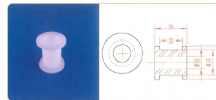
品名: Φ10轴套 规格: Φ10×26L 材质: UPE 编号: CT-ZT-011
