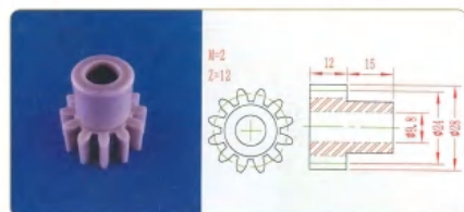
品名: 12齿24直齿轮 材质: PP
