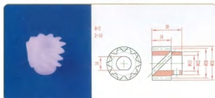
品名: 10齿螺旋齿轮 规格: M2×10Z×28L 材质: PVDF 编号: CT-LXCL-013
