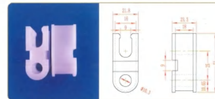
品名: 25插件 材质: PP
