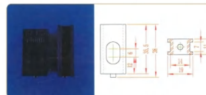
品名: 30上插件 材质: MC 规格: Φ10×37.5H 编号: CT-CX-007
