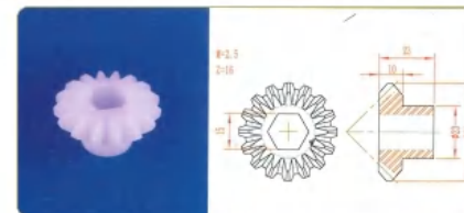
品名: 16齿伞齿轮 材质: PE
