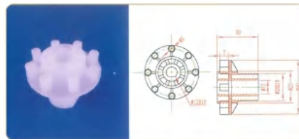
品名: 8齿钉齿轮 规格: 8Z×Φ40×30L 材质: PVDF 编号: CT-DCL-012
