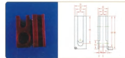
品名: 16.8插件 材质: 尼龙
