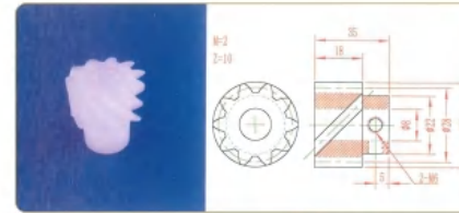
品名: 10齿螺旋齿轮 规格: M2×10Z×35L 材质: PVDF 编号: CT-LXCL-022
