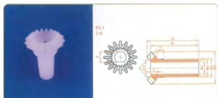
品名: 16齿伞齿轮 规格: M2.5×16Z×60L 材质: PVDF 编号: CT-SCL-033
