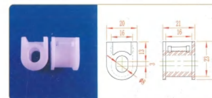
品名: 下插件 材质: UPE
