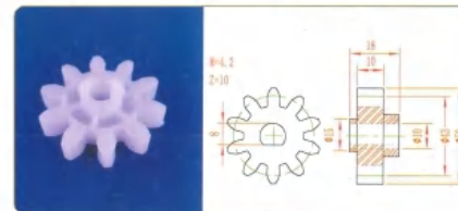
品名: 10齿43直齿轮 规格: M4.2×10Z 材质: PP 编号: CT-ZCL-076
