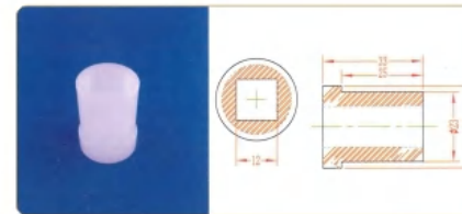
品名: 方12轴套 规格: 方孔12×33L 材质: PVDF 编号: CT-ZT-017
