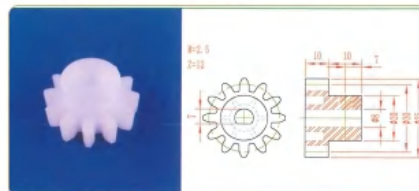
品名: 12齿30直齿轮 规格: M2.5×10Z 材质: PP 编号: CT-ZCL-026
