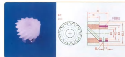
品名: 13齿40直齿轮 规格: M3×13Z 材质: PVDF 编号: CT-ZCL-063
