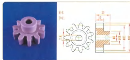
品名: 11齿33直齿轮 规格: M3×11Z 材质: PVC 编号: CT-ZCL-108
