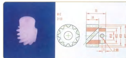
品名: 10齿螺旋齿轮 规格: M2×10Z×35L 材质: PVDF 编号: CT-LXCL-023
